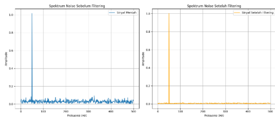
Gambar 2. Spektrum Noise Sebelum dan Sesudah Filtering
