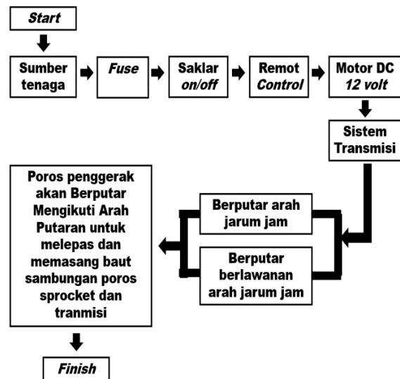
Gambar 3. Diagram kerja alat (Sumber : dibuat oleh peneliti)
